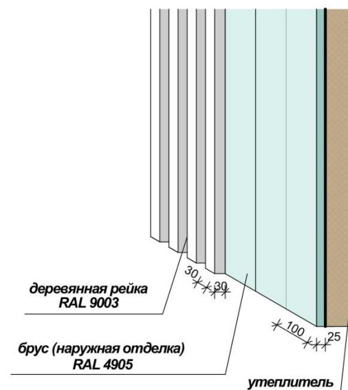
Примыкание декоративной рейки к наружной отделке фасада
