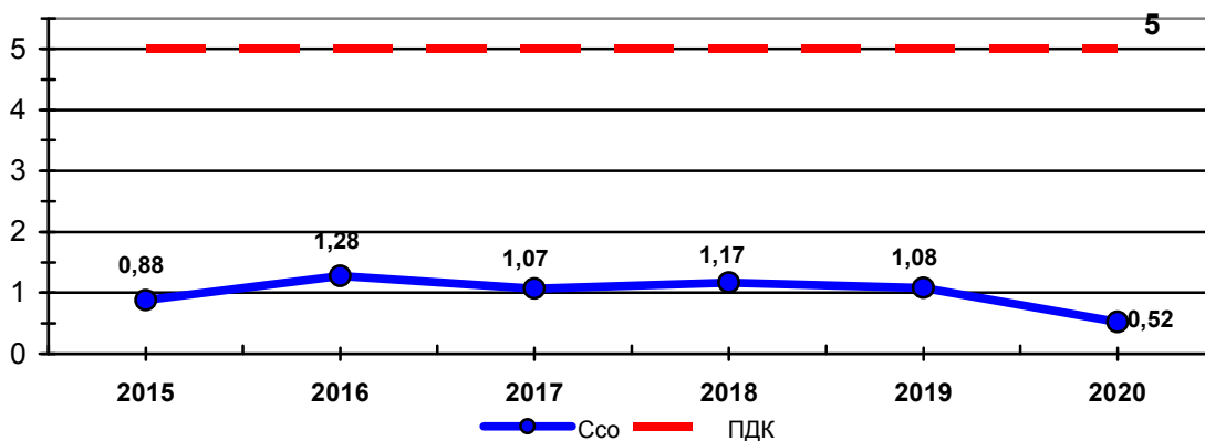
График 3 Средние концентрации оксида углерода в мг/м 3 (ПДК со =5 мг/м 3 ) на МП «Парк Победы» за 2015 - 2020 годы.
