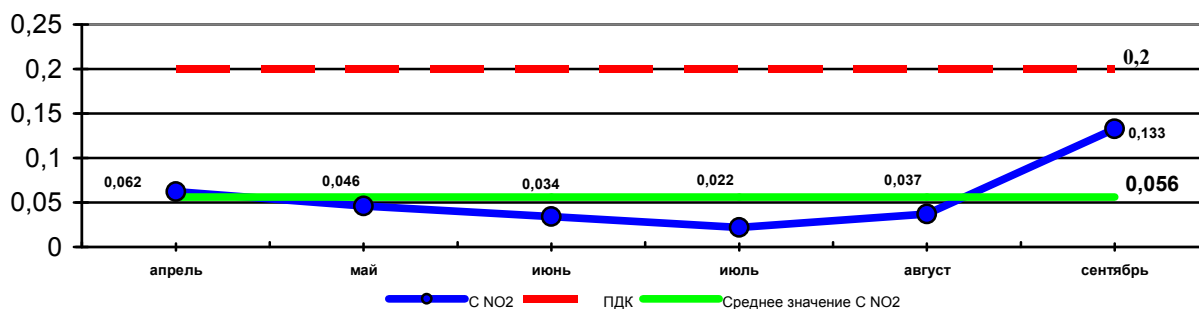
График 7 Динамика изменения средних концентраций диоксида азота в мг/м 3 (ПДК NO 2 =0,2 мг/м 3 ) на МП «Парк Победы» в 2020 году
