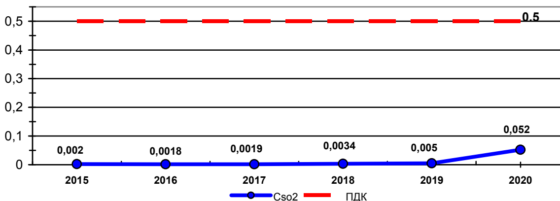
График 6 Средние концентрации диоксида серы (SO 2 ) (ПДК=0,5 мг/м 3 ) на МП «Парк Победы» за 2015 - 2020 годы.
