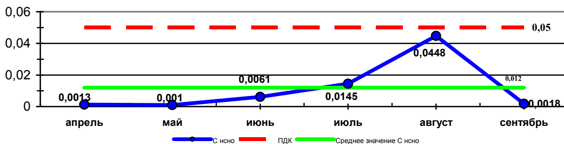
График 16 Динамика изменения средних концентраций формальдегида в \text{мг/м}^3 ( \text{ПДК}_{\text{НСНО}}=0,05 \text{ мг/м}^3 ) на МП «Парк Победы» в 2020 году
