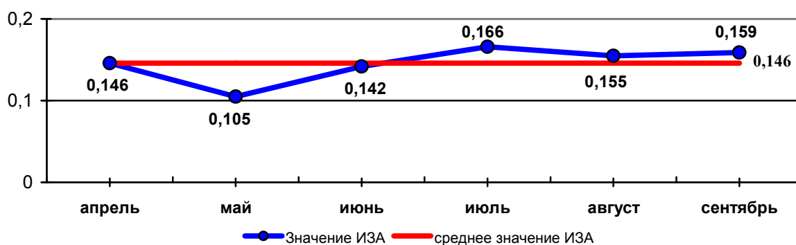
График 14 Динамика изменения ИЗА взвешенными частицами по месяцам на МП «Парк Победы» за 2020 год
