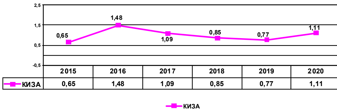
График 19 Сравнительная характеристика значений КИЗА на маршрутном посту «Парк Победы» за 2015 - 2020 годы.
