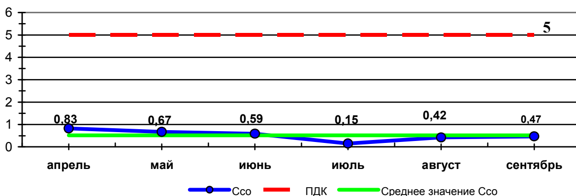
График 1 Динамика изменения средних концентраций оксида углерода в г. Йошкар-Оле за 2020 год
