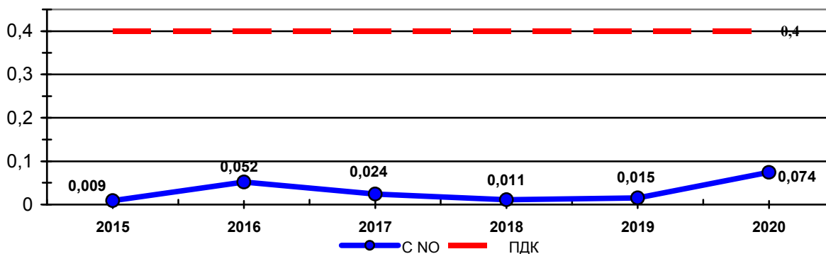
График 12 Средние концентрации оксида азота в мг/м 3 (ПДК NO =0,4 мг/м 3 ) на МП «Парк Победы» за 2015 - 2020 годы.
