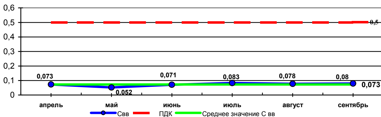
График 13 Динамика изменения средних концентраций взвешенных частиц в \text{мг/м}^3 (ПДК ВВ=0,5 \text{мг/м}^3 ) на МП «Парк Победы» в 2020 году
