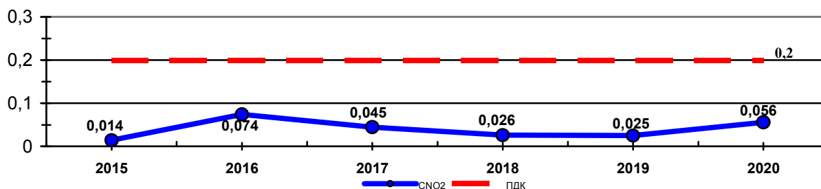
График 9 Средние концентрации диоксида азота в \text{мг/м}^3 (ПДК \text{NO}_2=0,2 \text{ мг/м}^3 ) на МП «Парк Победы» за 2015 - 2020 годы.
