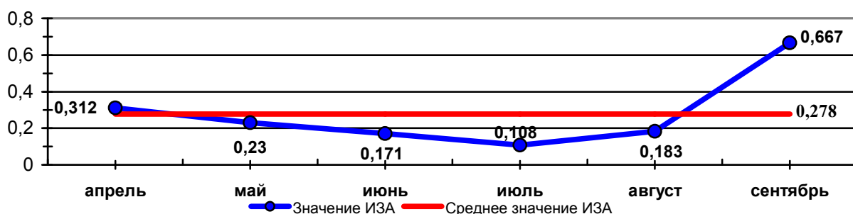
График 8 Динамика изменения ИЗА диоксидом азота по месяцам на МП «Парк Победы» за 2020 год
