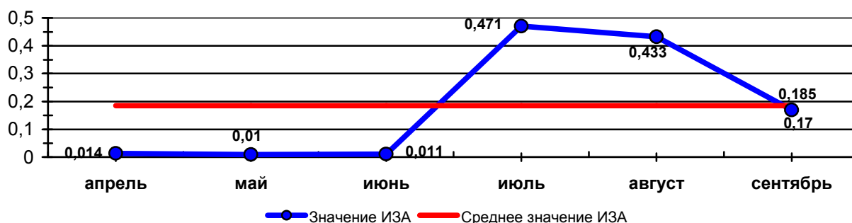
График 11 Динамика изменения ИЗА оксидом азота по месяцам на МП «Парк Победы» за 2020 год
