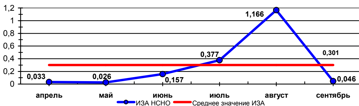
График 17 Динамика изменения ИЗА формальдегидом по месяцам на МП «Парк Победы» за 2020 год
