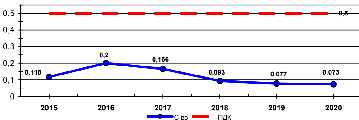
График 15 Средние концентрации взвешенных частиц в \text{мг/м}^3 (ПДК ВВ= 0,5 \text{ мг/м}^3 ) на МП «Парк Победы» за 2015 - 2020 годы.
