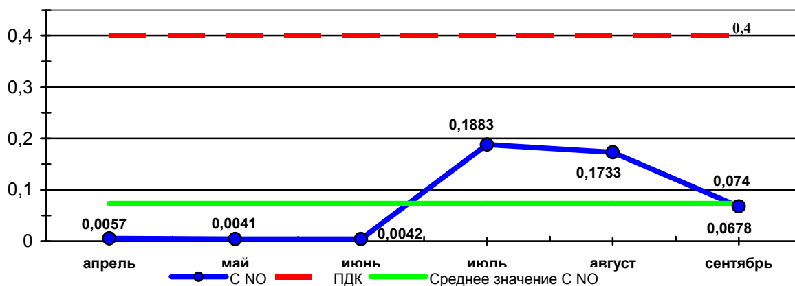
График 10 Динамика изменения средних концентраций оксида азота в мг/м 3 (ПДК NO=0,4 мг/м 3 ) на МП «Парк Победы» в 2020 году
