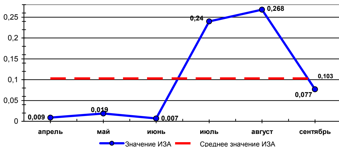
График 5 Динамика изменения ИЗА диоксидом серы по месяцам на МП «Парк Победы» за 2020 год
