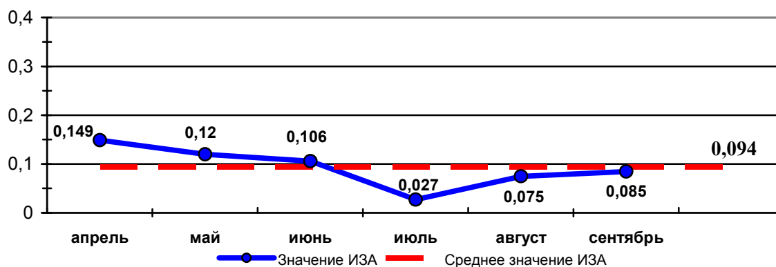
График 2 Динамика изменения ИЗА оксидом углерода по месяцам на МП «Парк Победы» за 2020 год
