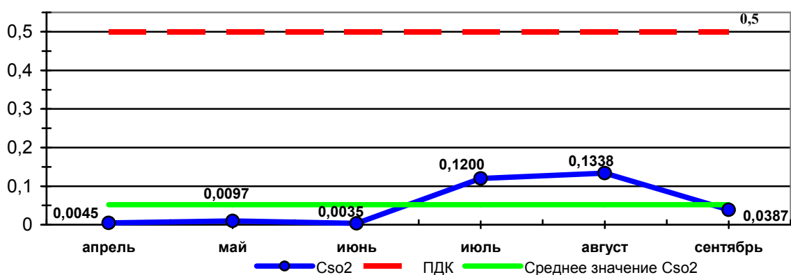
График 4 Динамика изменения средних концентраций диоксида серы в мг/м 3 (ПДК SO 2 =0,5 мг/м 3 ) на МП «Парк Победы» за 2020 год
