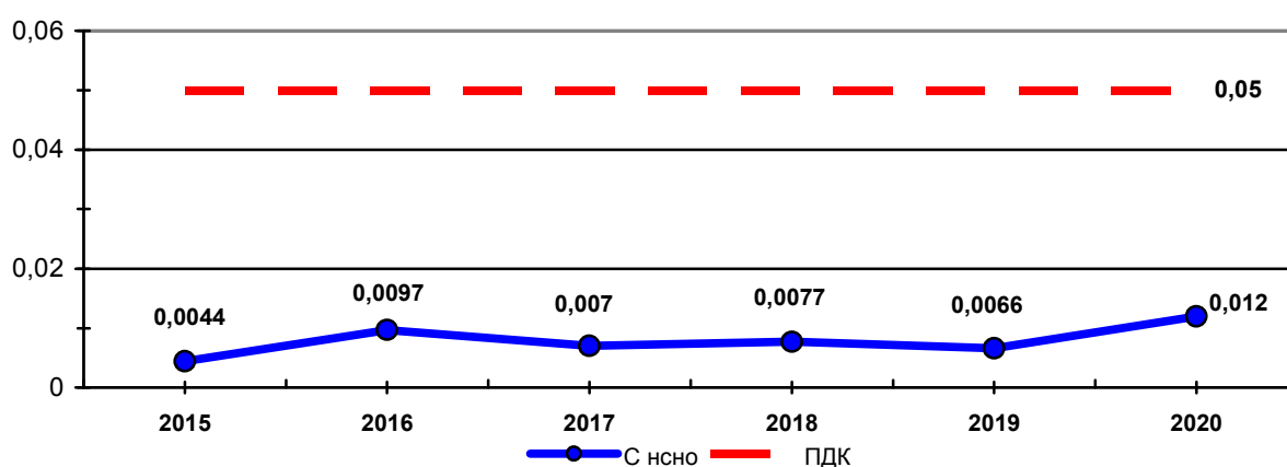
График 18 Средние концентрации формальдегида в мг/м 3 (ПДКнсно=0,05 мг/м 3 ) на МП «Парк Победы» за 2015 - 2020 годы.
