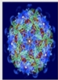
Вирус ящура
