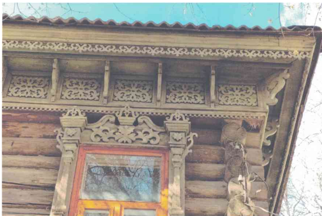
Фото 11. ОКН «Дом с деревянной резьбой». Фрагмент главного (северо-восточного) фасада. Следы увлажнения и загнивание древесины в чашках соединения бревен, под оконными проемами, в карнизной части; поражение древесины жучком, водосточные желоба, трубы и водосборные воронки утрачены.
