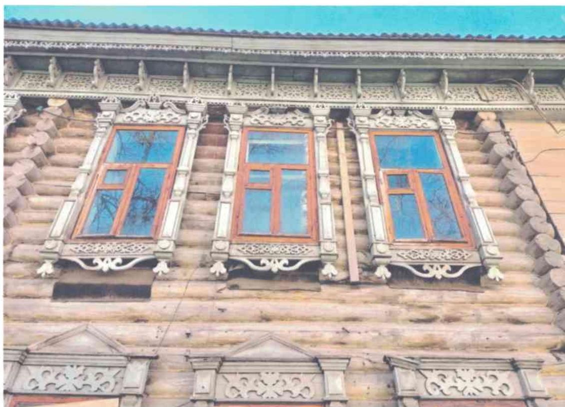
Фото 9. ОКН «Дом с деревянной резьбой». Фрагмент главного (северо-восточного) фасада. Износ и потеря прочности древесины, следы увлажнения и загнивание древесины под оконными проемами, в карнизной части; поражение древесины жучком.
