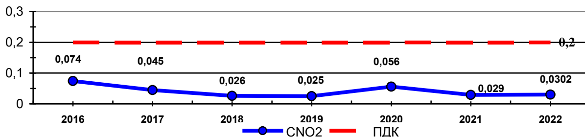
График 9 Средние концентрации диоксида азота в мг/м 3 (ПДК NO 2 =0,2 мг/м 3 ) на МП «Парк Победы» за 2016 – 2022 годы.
