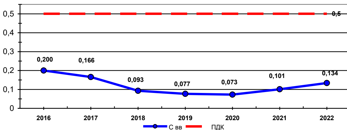
График 15 Средние концентрации взвешенных частиц в мг/м 3 (ПДК вв=0,5 мг/м 3 ) на МП «Парк Победы» за 2016 - 2022 годы.
