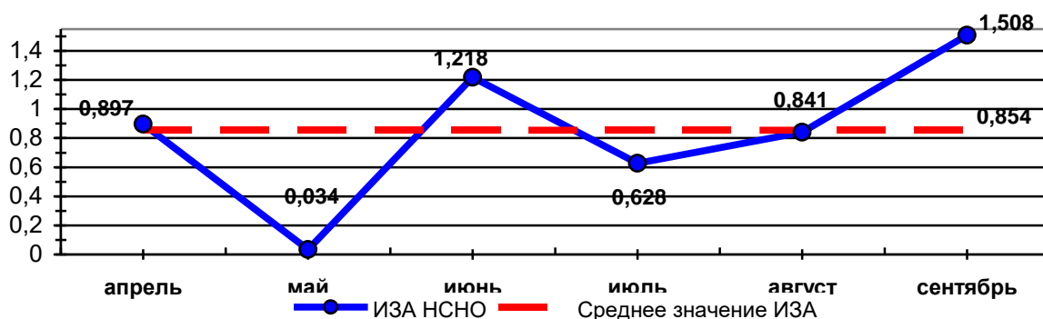
График 17 Динамика изменения ИЗА формальдегидом по месяцам на МП «Парк Победы» за 2022 год
