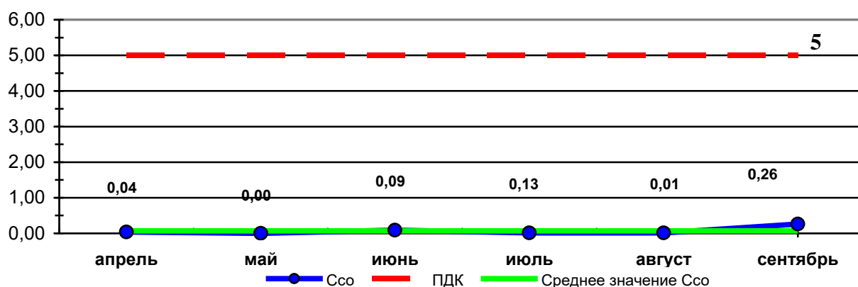
График 1 Динамика изменения средних концентраций оксида углерода в г. Йошкар-Оле за 2022 год
