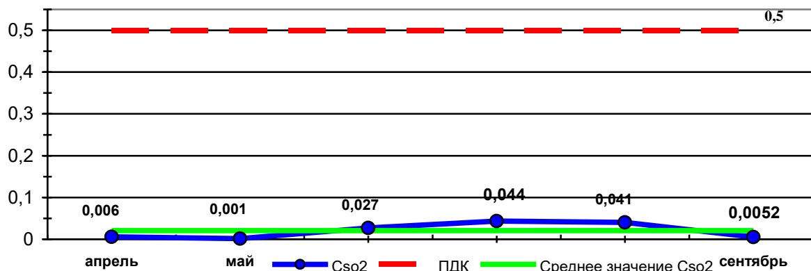
График 4 Динамика изменения средних концентраций диоксида серы в \text{мг/м}^3 ( SO_2 ПДК=0,5 \text{мг/м}^3 ) на МП «Парк Победы» за 2022 год
