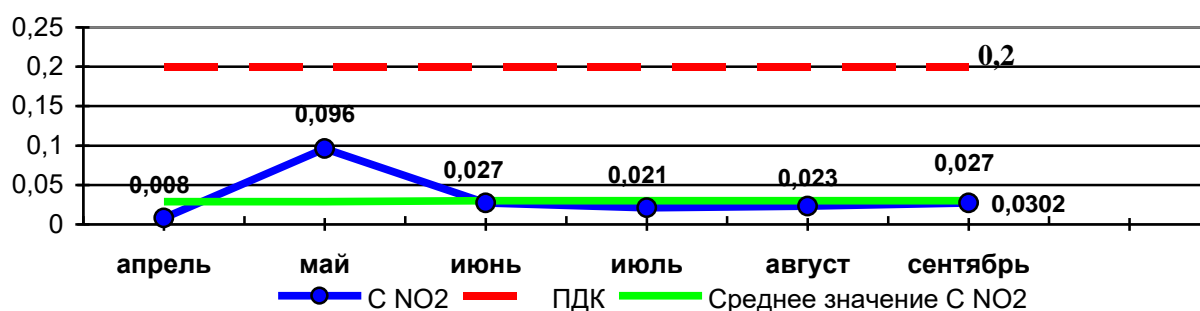
График 7 Динамика изменения средних концентраций диоксида азота в мг/м 3 (ПДК NO 2 =0,2 мг/м 3 ) на МП «Парк Победы» в 2022 году
