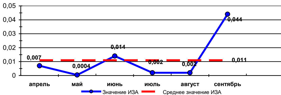
График 2 Динамика изменения ИЗА оксидом углерода по месяцам на МП «Парк Победы» за 2022 год
