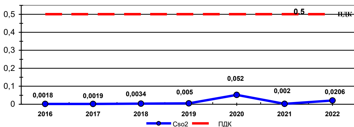
График 6 Средние концентрации диоксида серы (SO 2 ) (ПДК=0,5 мг/м 3 ) на МП «Парк Победы» за 2016-2022 годы.
