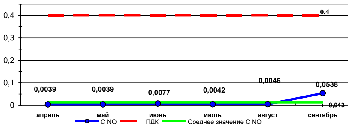
График 10 Динамика изменения средних концентраций оксида азота в мг/м 3 (ПДК NO=0,4 мг/м 3 ) на МП «Парк Победы» в 2022 году
