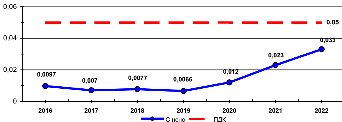
График 18 Средние концентрации формальдегида в мг/м 3 (ПДКнсно=0,05 мг/м 3 ) на МП «Парк Победы» за 2016 - 2022 годы.
