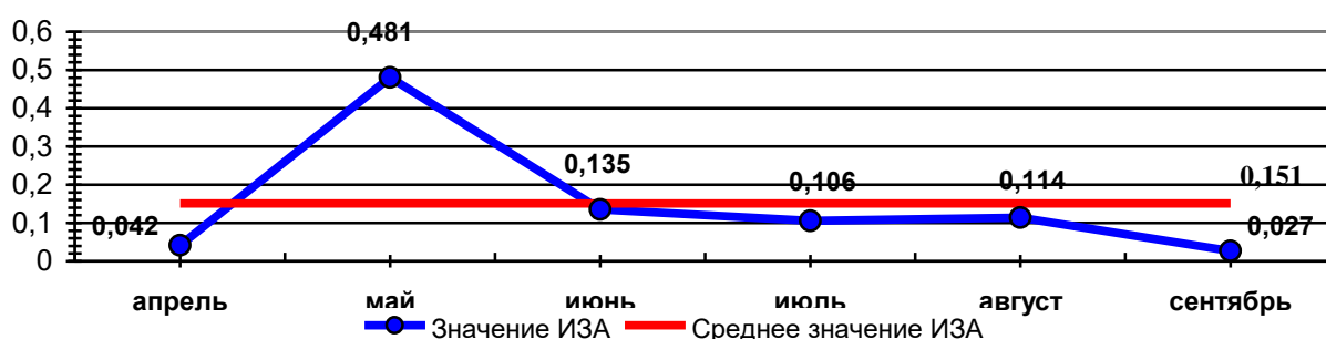
График 8 Динамика изменения ИЗА диоксидом азота по месяцам на МП «Парк Победы» за 2022 год
