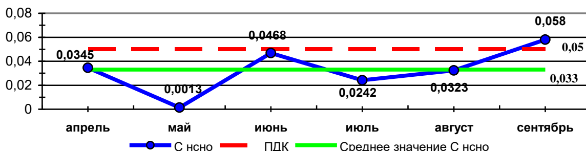
График 16 Динамика изменения средних концентраций формальдегида в мг/м 3 (ПДК HCHO =0,05 мг/м 3 ) на МП «Парк Победы» в 2022 году
