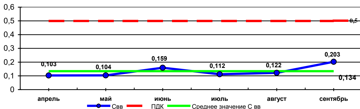
График 13 Динамика изменения средних концентраций взвешенных частиц в мг/м 3 (ПДК ВВ=0,5 мг/м 3 ) на МП «Парк Победы» в 2022 году
