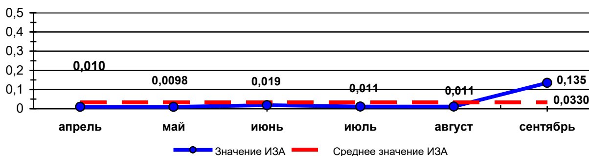
График 11 Динамика изменения ИЗА оксидом азота по месяцам на МП «Парк Победы» за 2022 год
