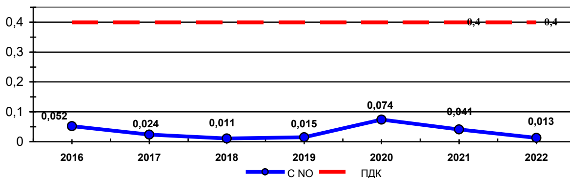
График 12 Средние концентрации оксида азота в мг/м 3 (ПДК NO=0,4 мг/м 3 ) на МП «Парк Победы» за 2016 - 2022 годы.
