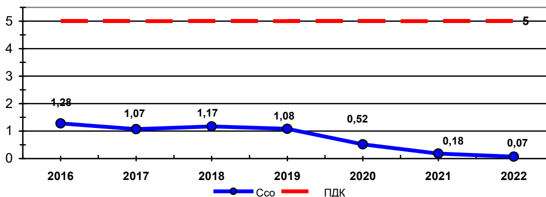
График 3 Средние концентрации оксида углерода в мг/м 3 (ПДК со =5 мг/м 3 ) на МП «Парк Победы» за 2016 - 2022 годы.
