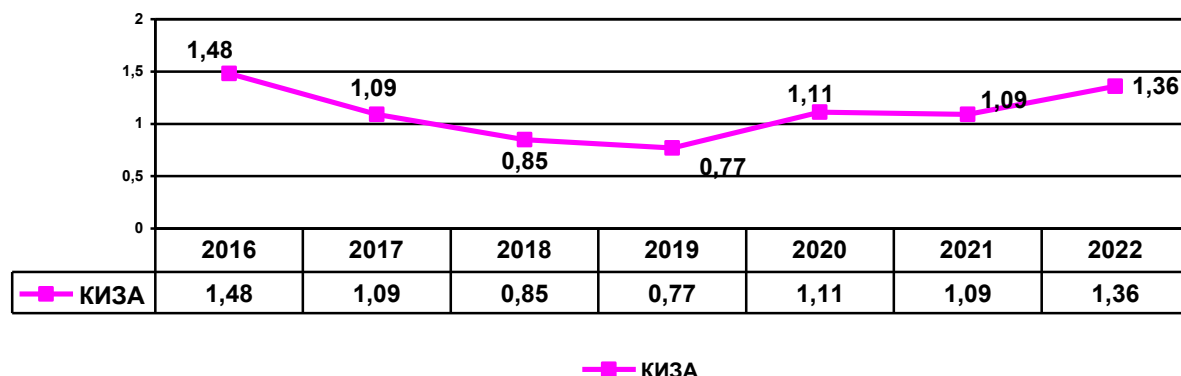
График 19 Сравнительная характеристика значений КИЗА на маршрутном посту «Парк Победы» за 2016 - 2022 годы.
