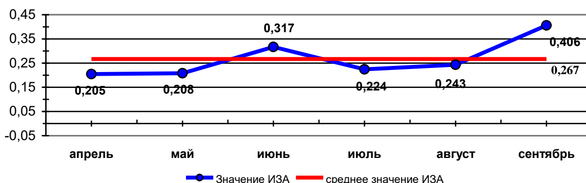
График 14 Динамика изменения ИЗА взвешенными частицами по месяцам на МП «Парк Победы» за 2022 год
