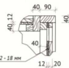
Узел 4
