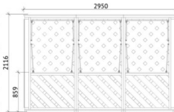
Лицевой фасад.
