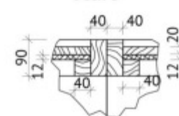
Узел 3
