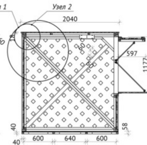
Разрез А-А.
