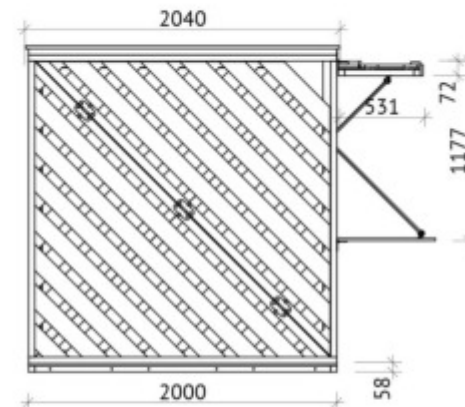
Боковой фасад.
