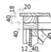
Узел 2
