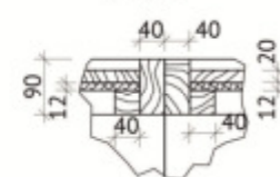
Узел 3
