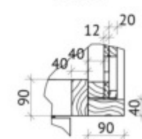
Узел 5
