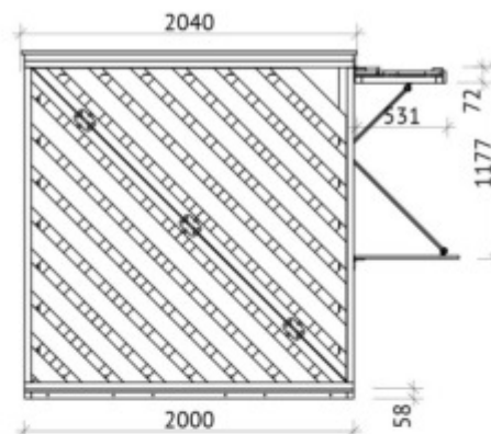
Боковой фасад.
