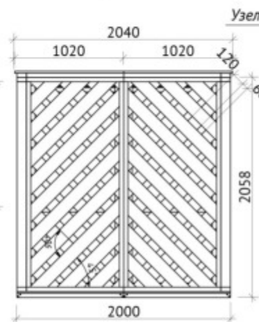
Задний фасад.
