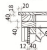
Узел 2
