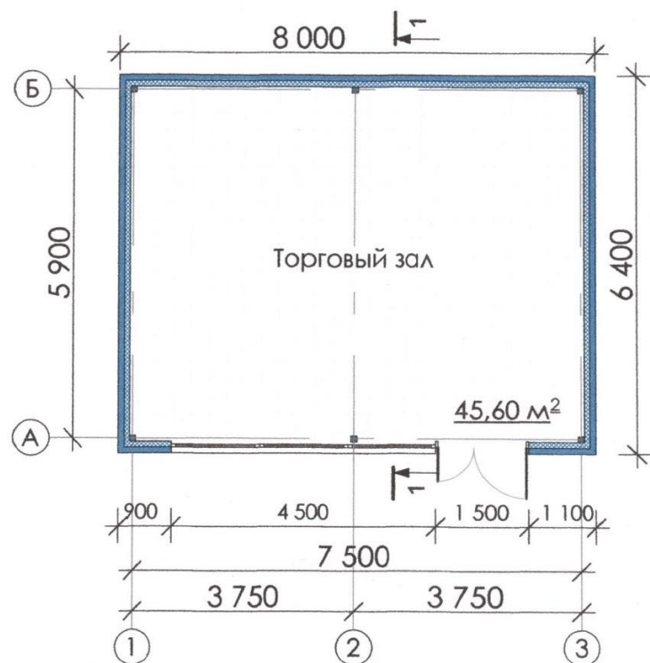
План этажа М1:100
