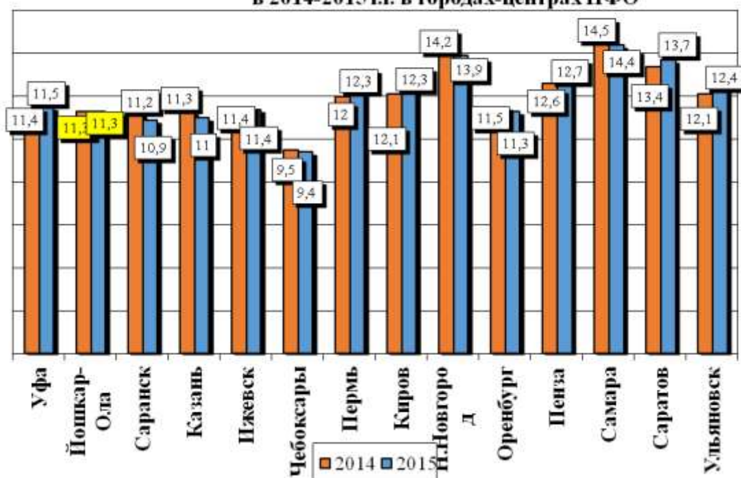
Умершие на 1000 населения, промилле, в 2014-2015 гг. в городах-центрах ПФО
