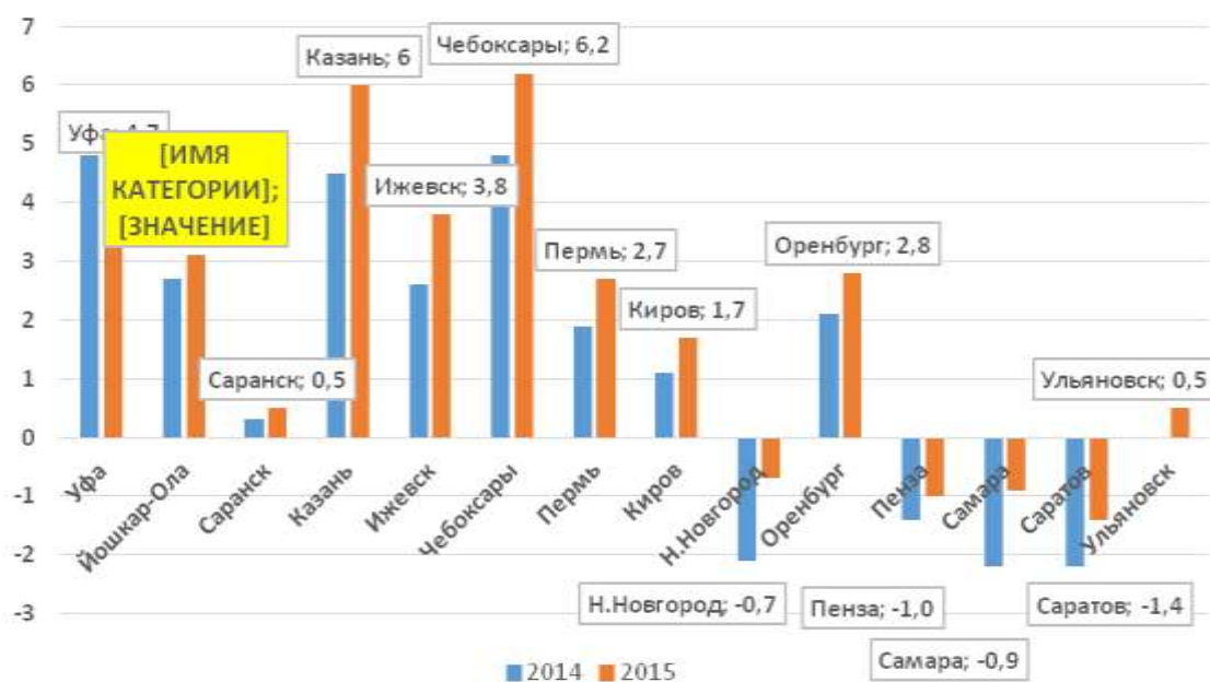
Естественный прирост (+), убыль (-) на 1000 населения, промилле в 2014-2015 г.г. в городах-центрах ПФО
