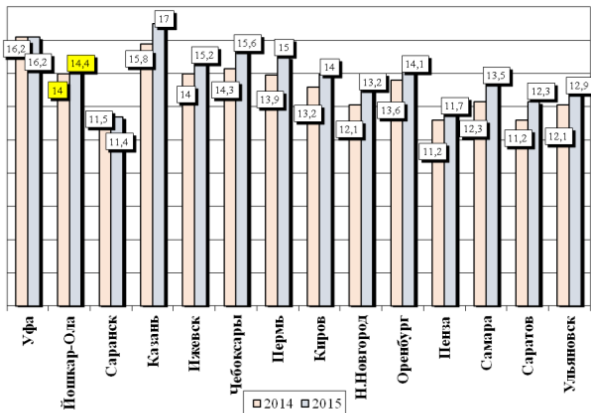
Родившиеся на 1000 населения, промилле, в 2014-2015 гг. по городам-центрам ПФО
