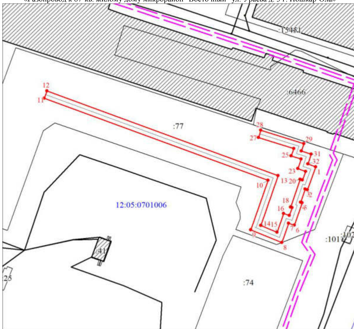
Схема расположения границ публичного сервитута «Газопровод к 87-кв. жилому дому микрорайон "Восточный" ул. Ураева д. 3 г. Йошкар-Ола»
