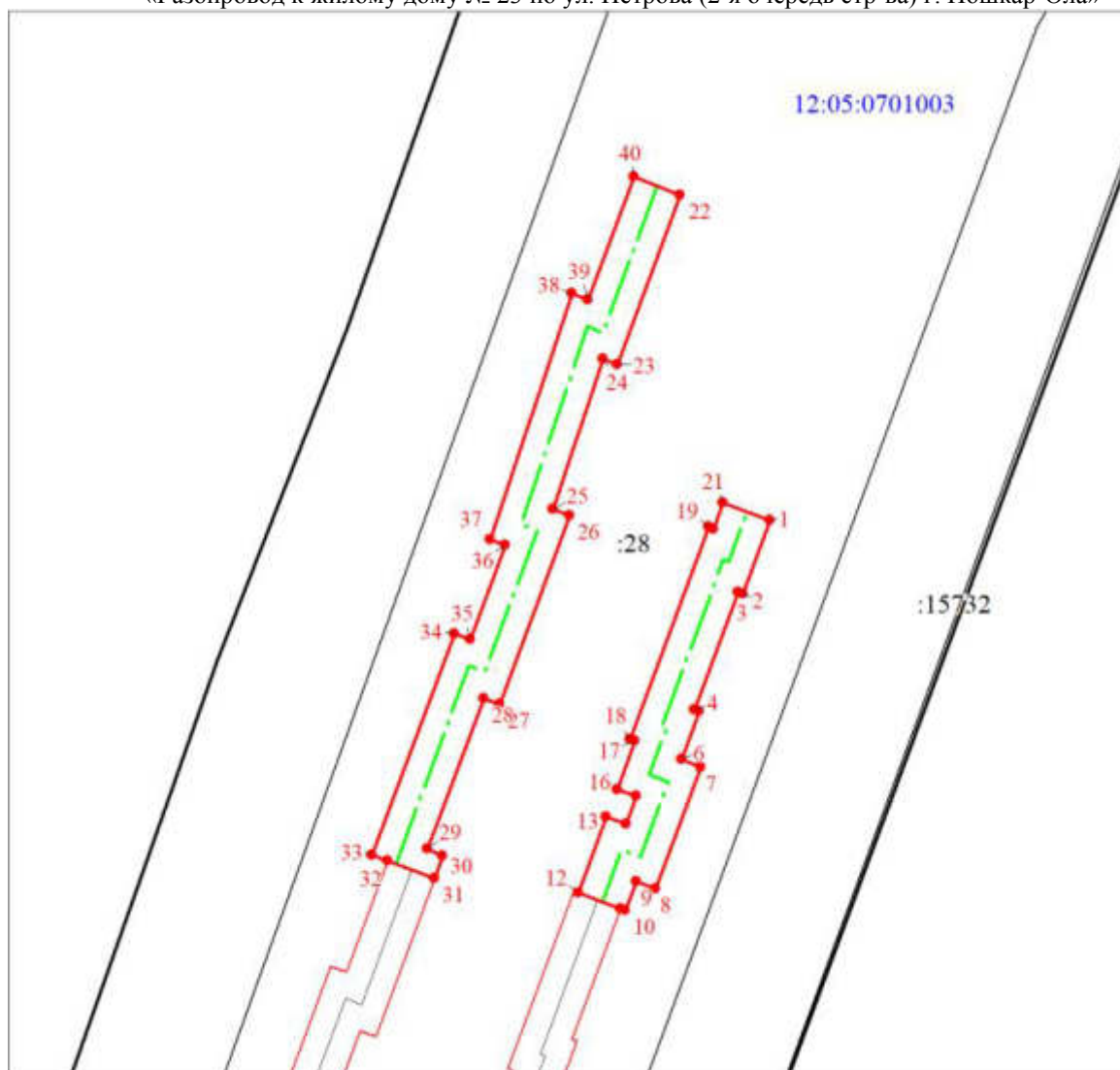
Схема расположения границ публичного сервитута «Газопровод к жилому дому № 23 по ул. Петрова (2-я очередь стр-ва) г. Йошкар-Ола»
